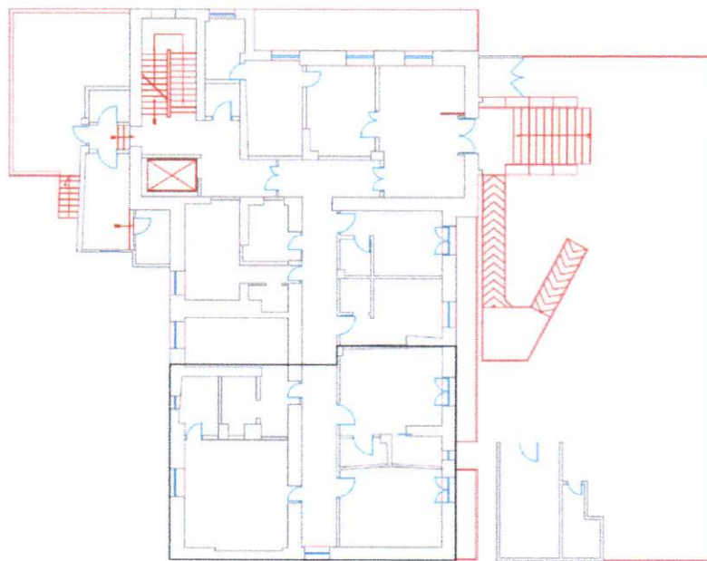
PLANIMETRIA PIANO RIALZATO STATO DEI LUOGHI
