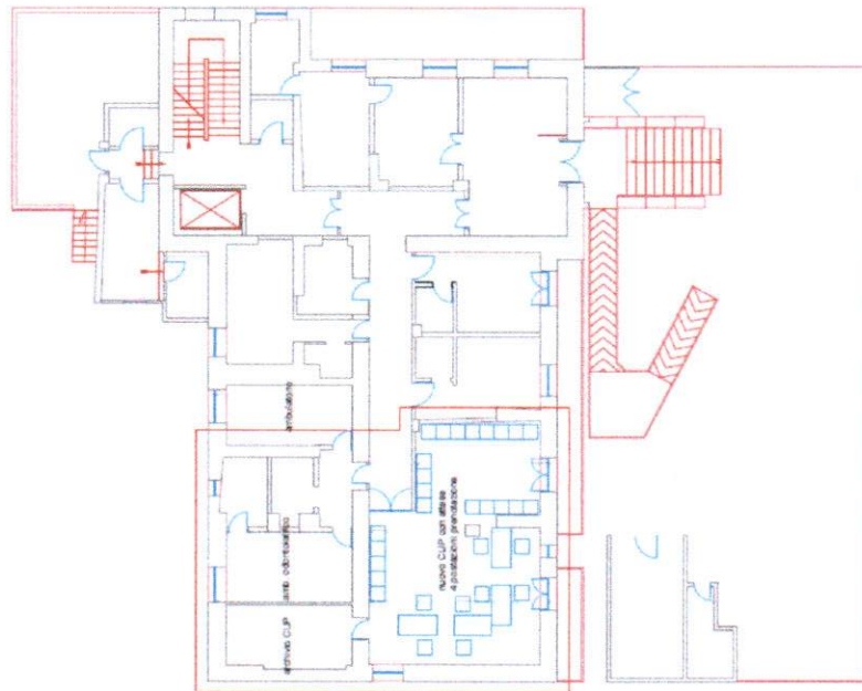
PLANIMETRIA PIANO RIALZATO STATO DI PROGETTO
